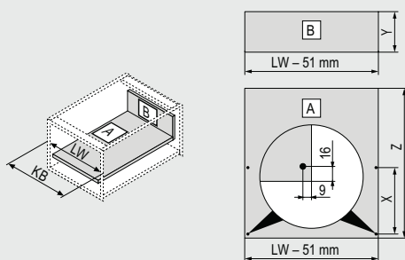
Débords pour panneaux agglo de 16 mm
